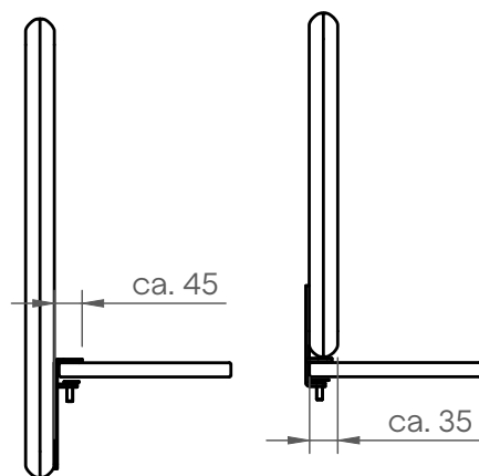
Hinter-Tisch-Montage
